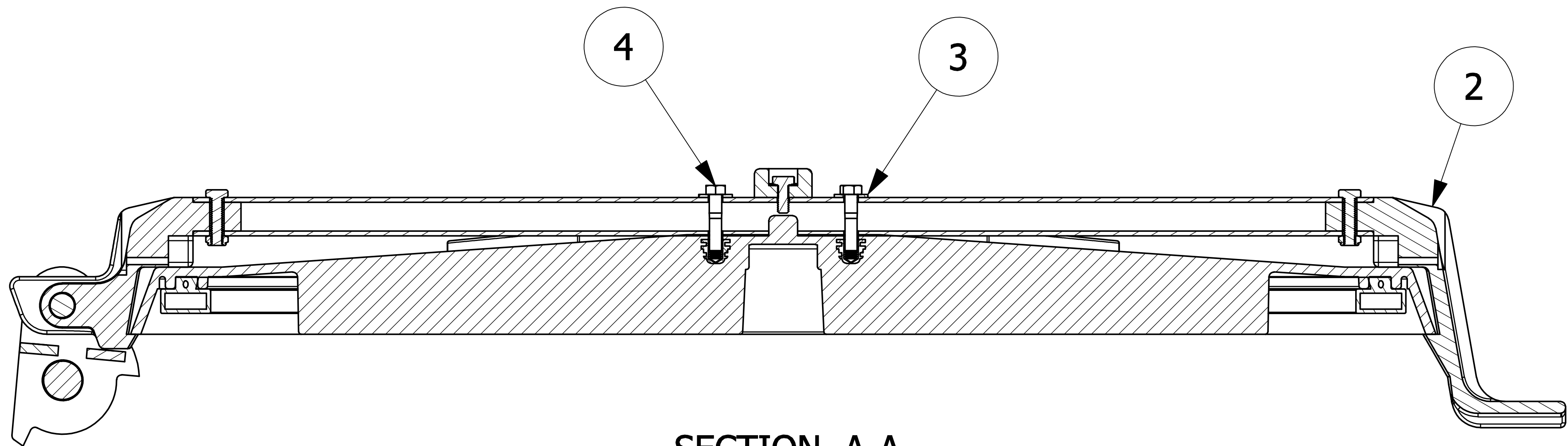
SECTION A-A
