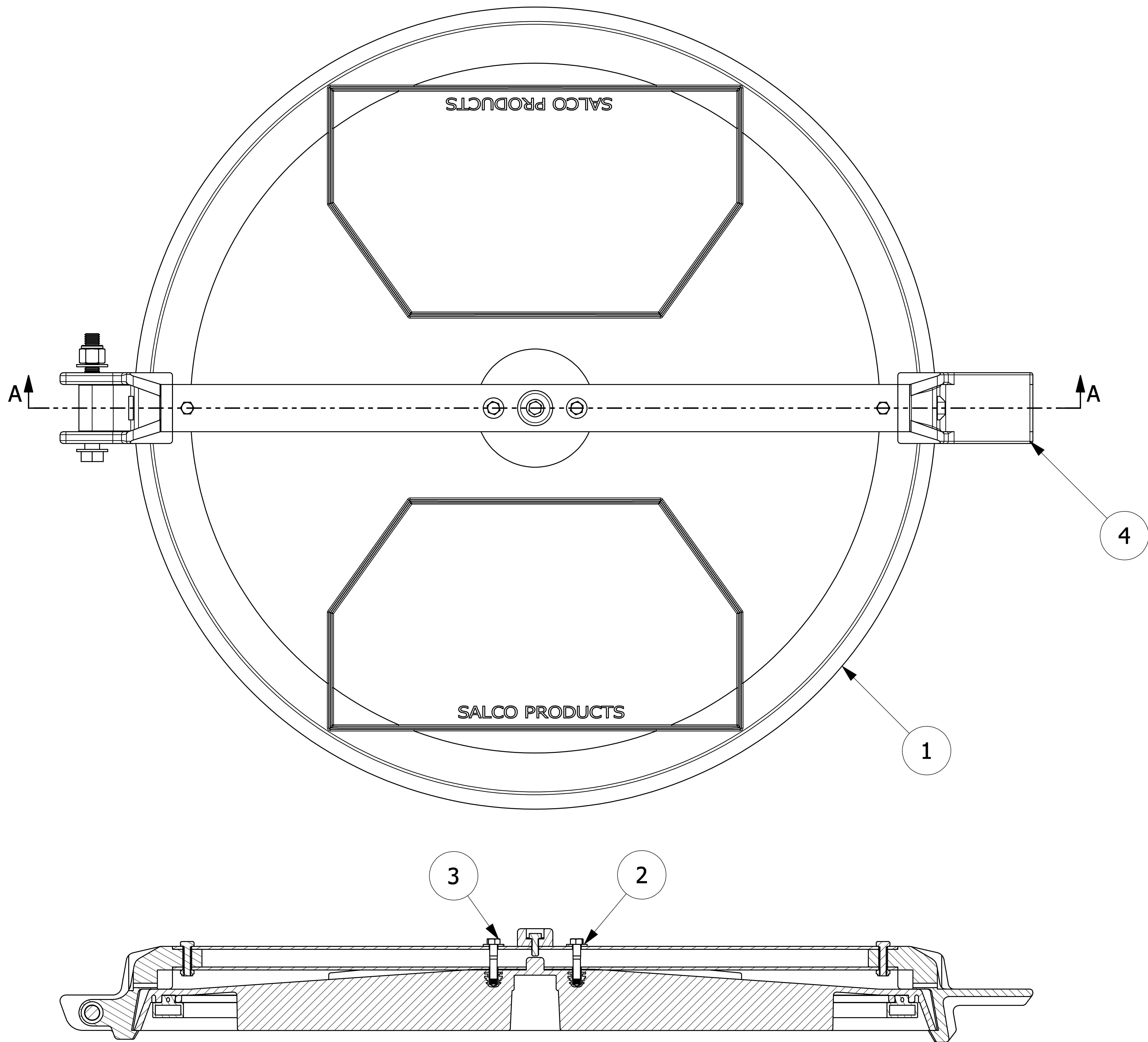
SECTION A-A
