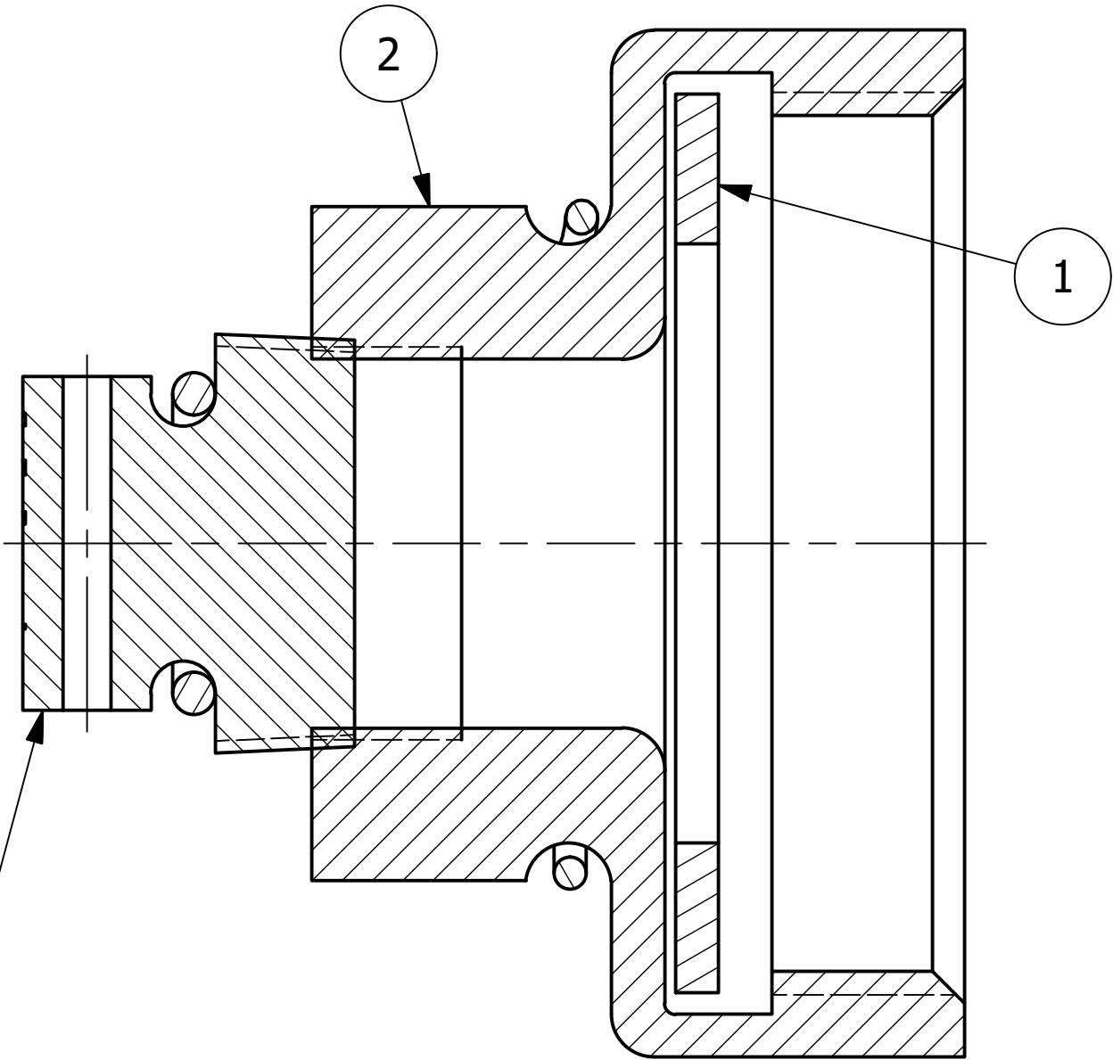
SECTION A-A
