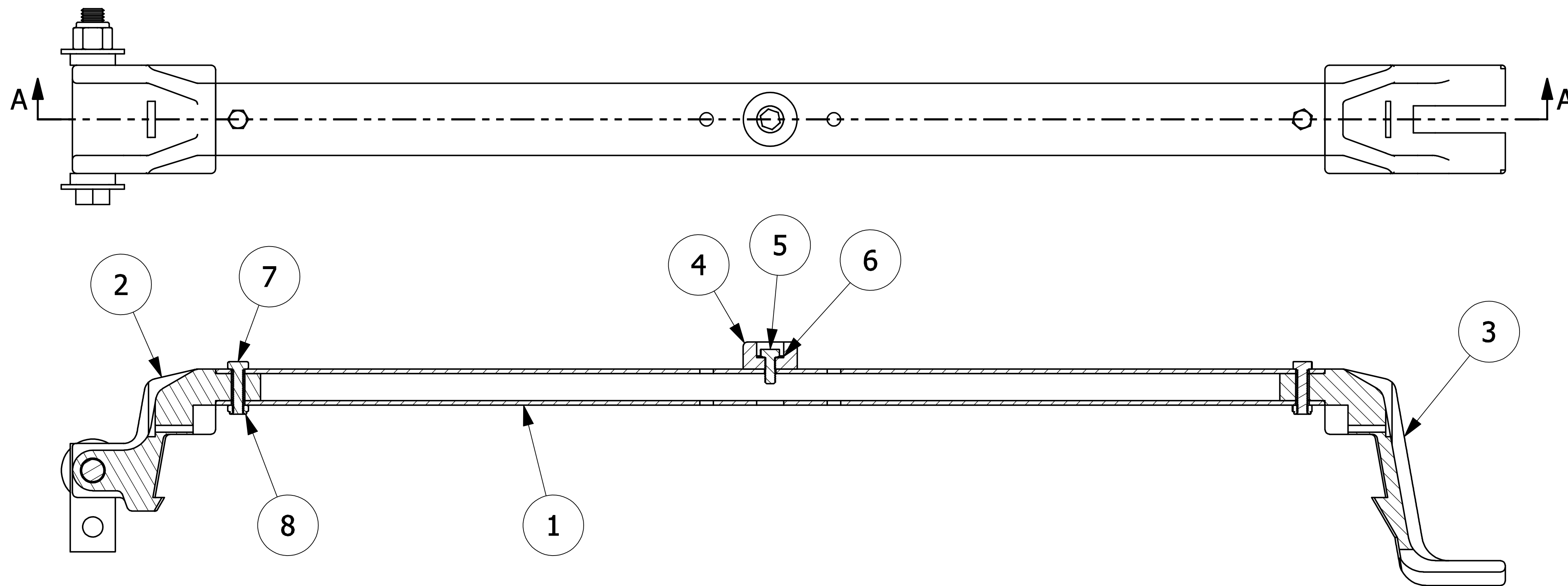
SECTION A-A
