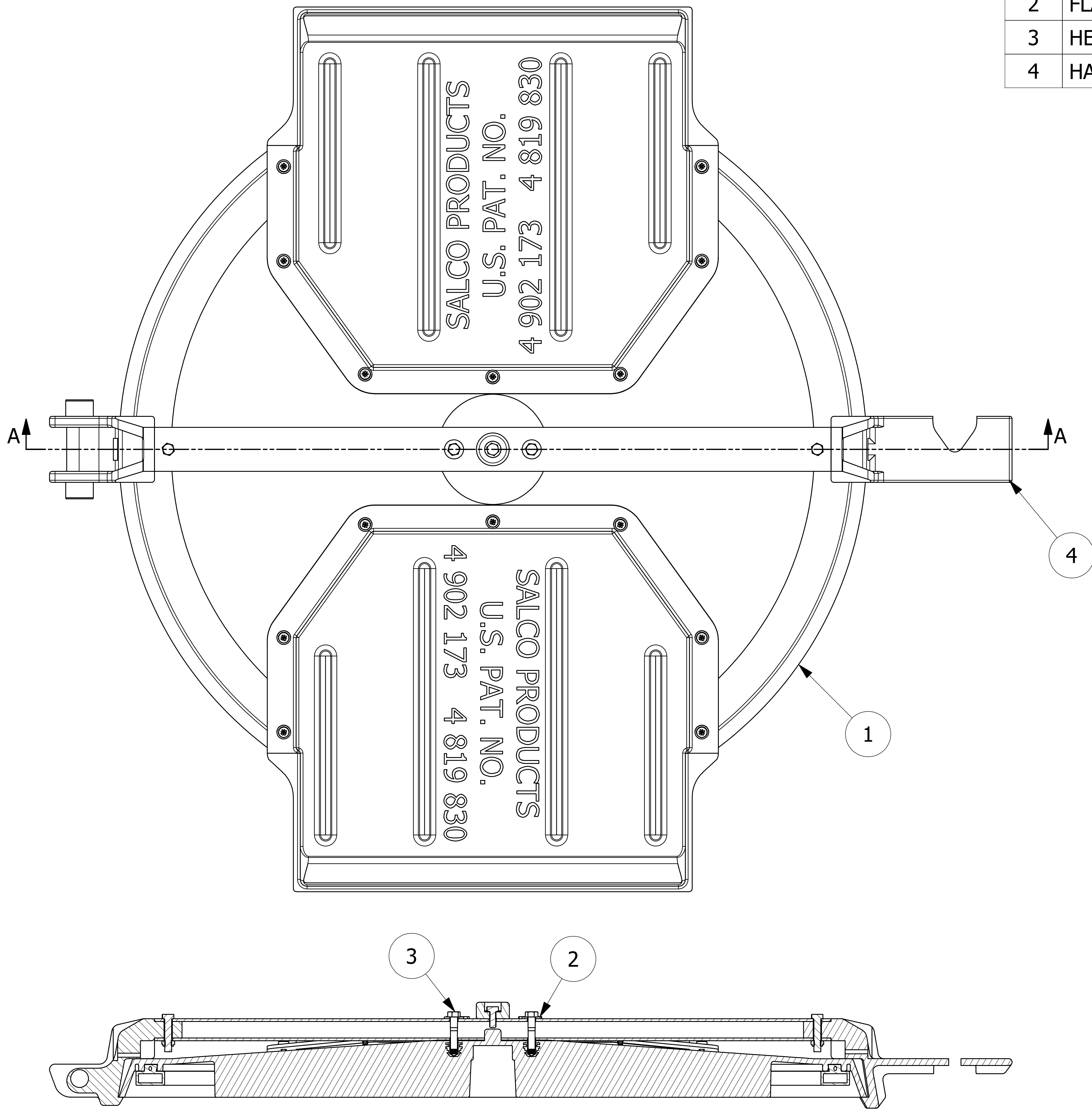
SECTION A-A
