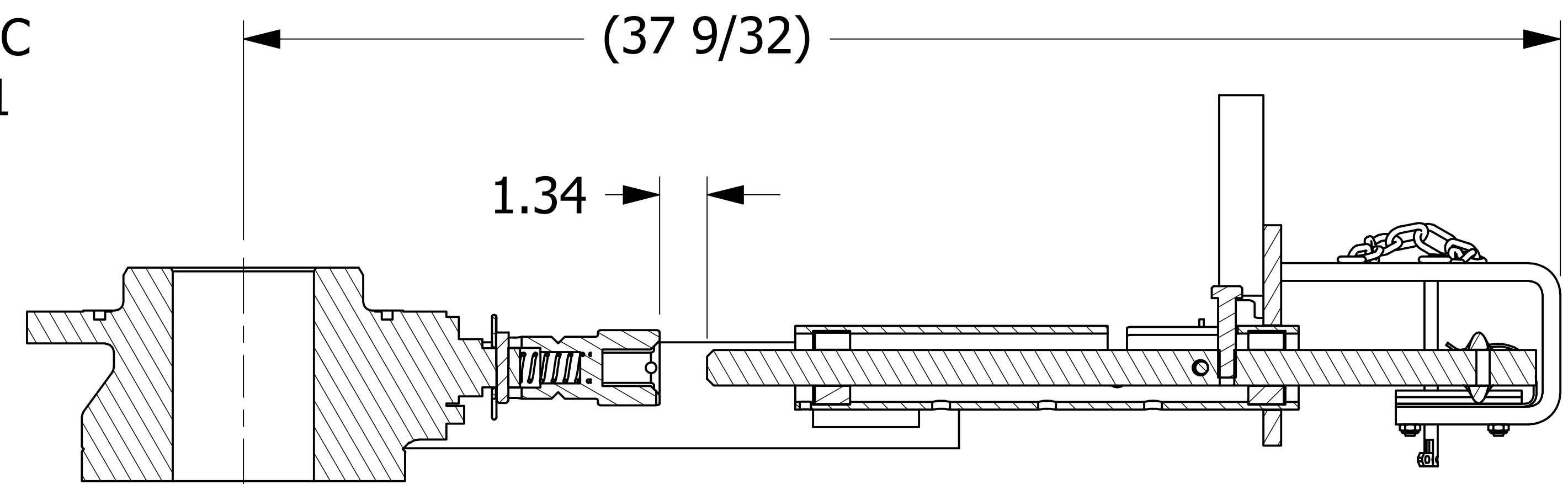
SECTION A-A SCALE 1:2
